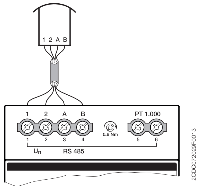
Anschlussbild
